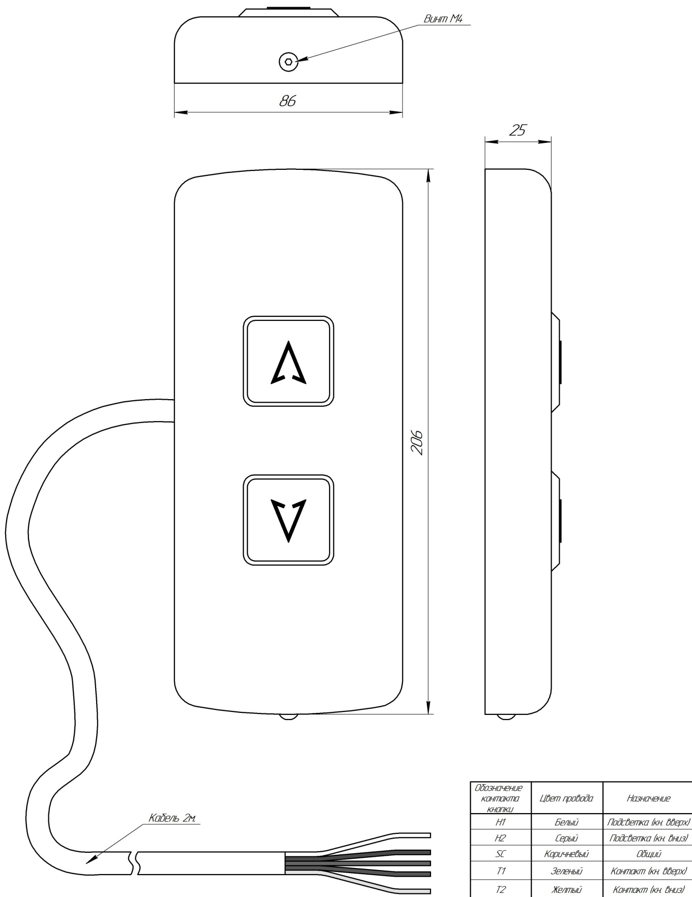
Рис.1 Внешний вид, габаритные и установочные размеры Вызывного поста ВП-2003-02
